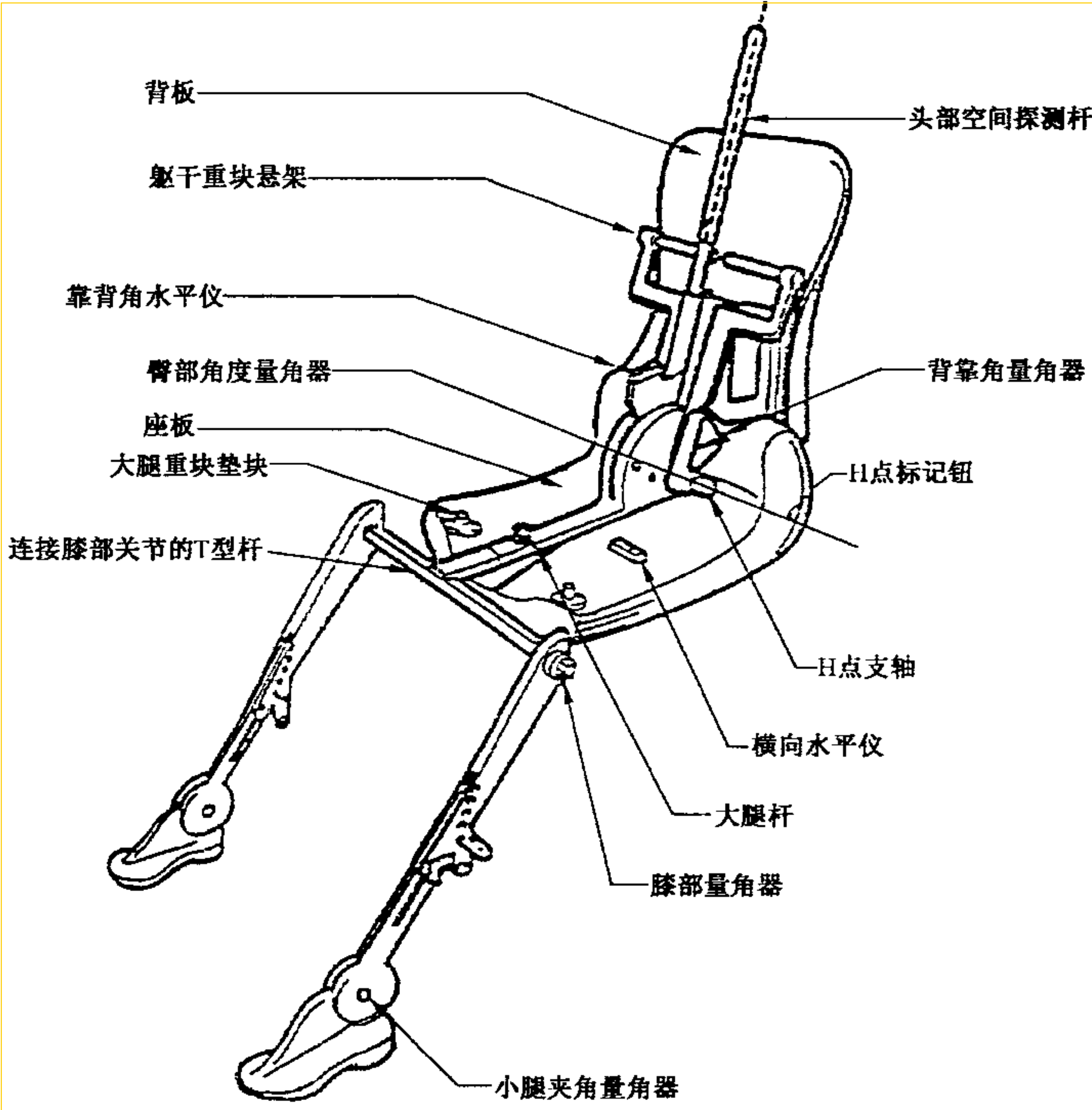
图 A.1 3-D H 装置构件名称
