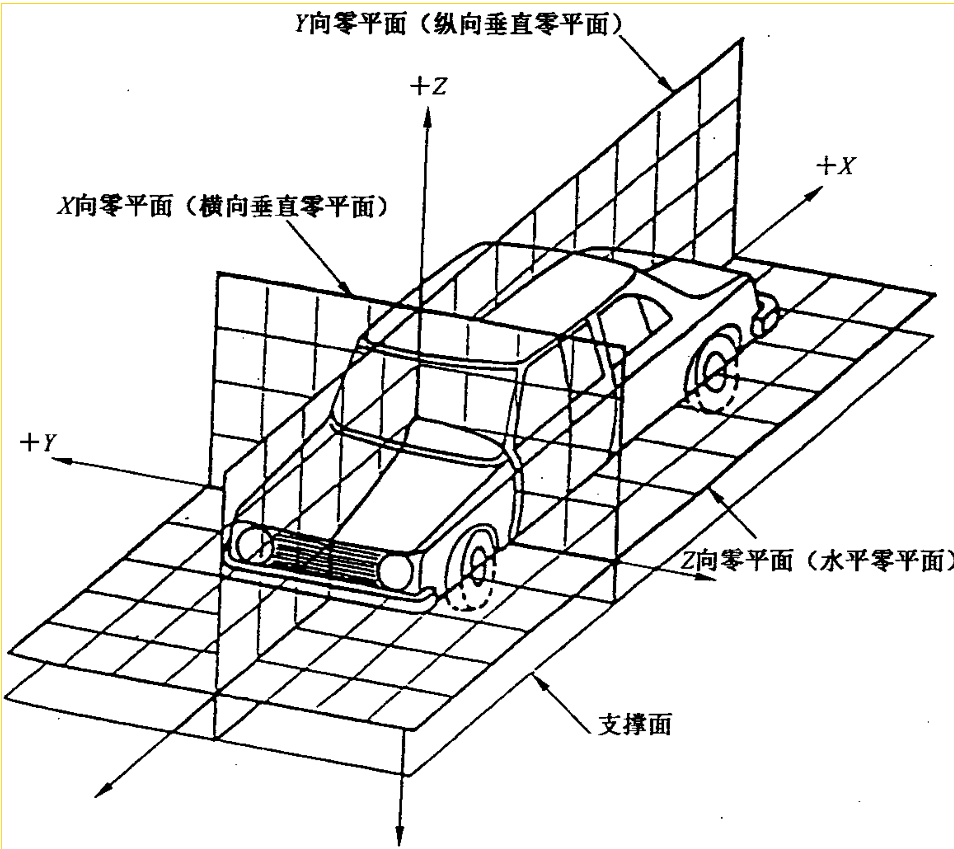
图 A.3 三维坐标系
