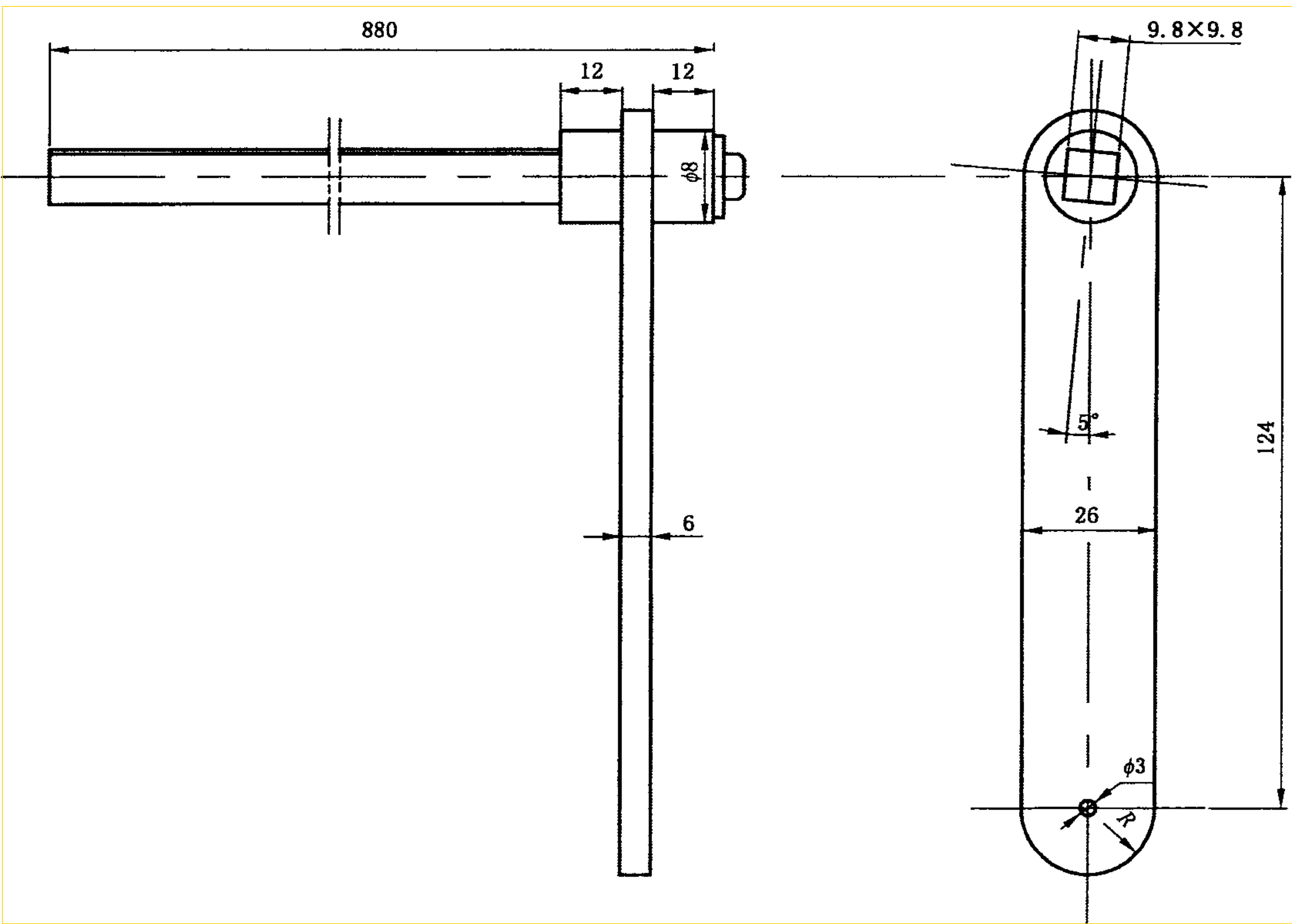
图 C.1 骨盆角度量规
